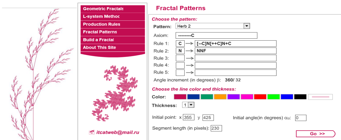
18. ábra: Egy fraktálnövény és L-system generáló képernyőmásolata
