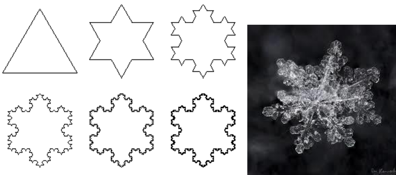
11. ábra: a Koch-görbe (hópehely) generálási lépései és egy valódi hópehely
