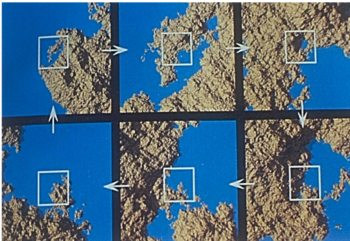
1. ábra: tengerpart önhasonló tulajdonsága
