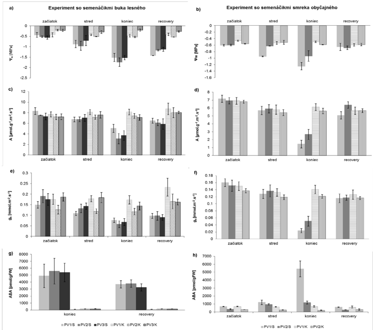
Graf a), b): Priebeh hodnôt vodného potenciálu asimilačných orgánov buka/smreka; c), d) priebeh hodnôt rýchlosti asimilácie CO 2 ; e), f) priebeh hodnôt stomatálnej vodivosti; g), h) priebeh hodnôt koncentrácie ABA v asimilačných orgánov buka lesného/smreka obyčajného počas experimentu. S označuje skupinu suchom stresovaných jedincov, K skupinu kontrolných jedincov. Chybové úsečky predstavujú strednú chybu.
