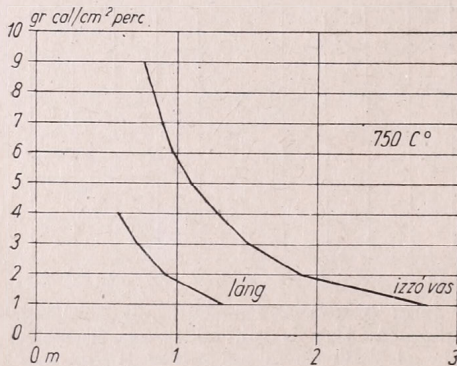
2. ábra. 750\text{ C}^\circ hőmérsékletű edzőkemence 100 \times 50\text{ cm} ajtónyílásán át kisugárzó hő alakulása az ajtótól különböző távolságban
